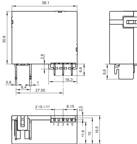
HFE66-4单线圈有1、5脚；HFE66-4双线圈有1、3、5脚。
