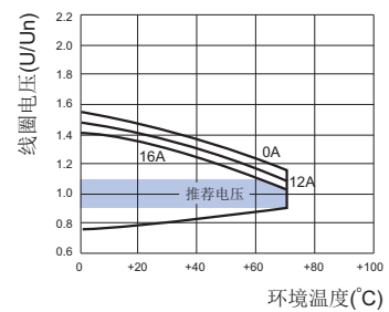
线圈工作温度曲线 (AC) *
