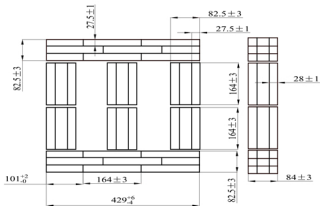
典型装配模式图
